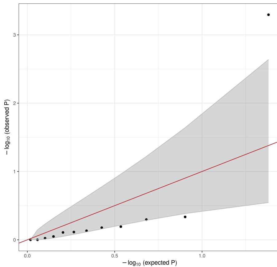
Intron Jaccard Index Q-Q plot: chr19:7592515-7592749:* ( MCOLN1 ; row ind
